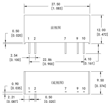
封装尺寸图
